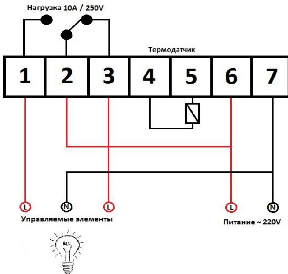
Схема подключения терморегулятора Ringder RC-112E 10A
